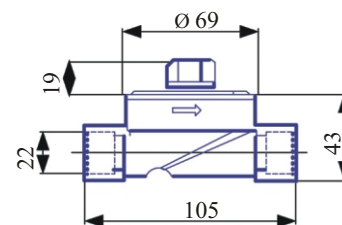
Рис.3 EAS для монтажа пайкой
