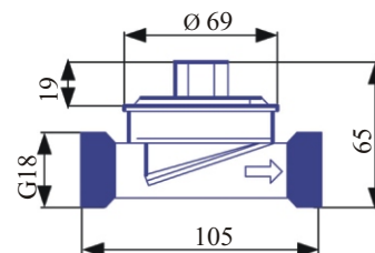
Рис.1 EAS с внешней резьбой
