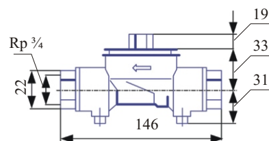
Рис.3 EAS с шаровыми кранами
