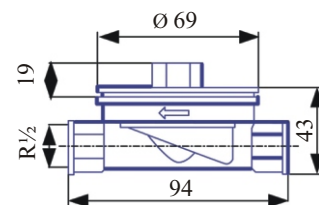
Рис.2 EAS с внутренней резьбой
